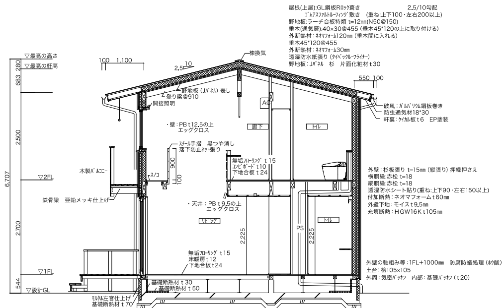
矩計図
